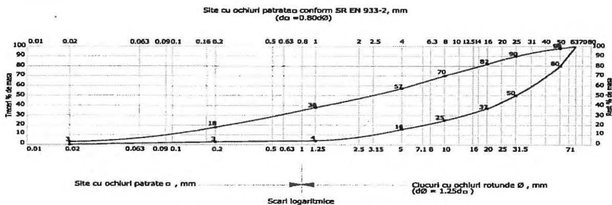
Figura 1 - Zona granulometrică prescrisă pentru balastul din stratul interior de fundație
